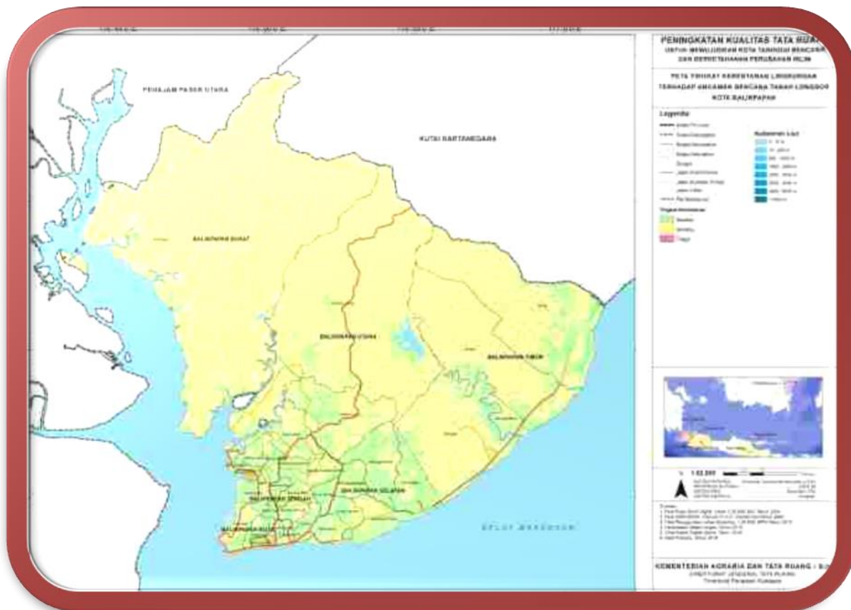
Peta 3. Tingkat Kerentanan Lingkungan Berdasarkan Ancaman Longsor Kota Balikpapan
